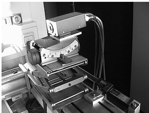
Bild 4: Messstand.
